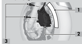
LADO DIREITO
